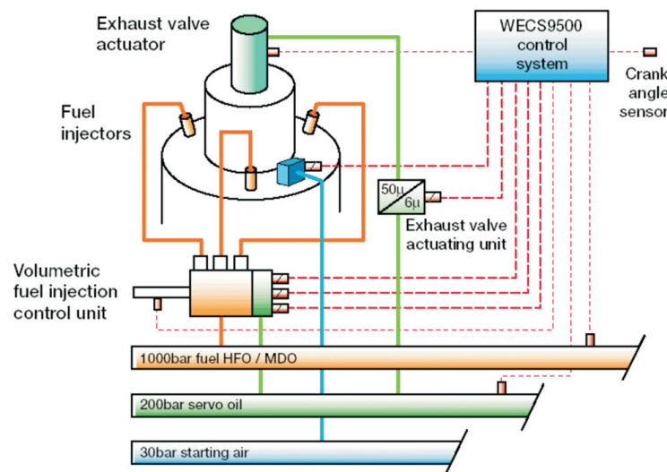
Rys. 7. Schemat funkcjonalny układu elektronicznego sterowania pracą silnika
